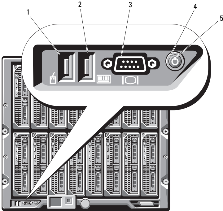
그림 1-4. 제어판 기능
